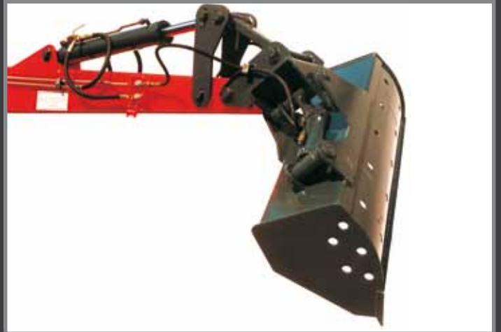
Schwenkbarer Grabenlöffel, 2 x 45°
